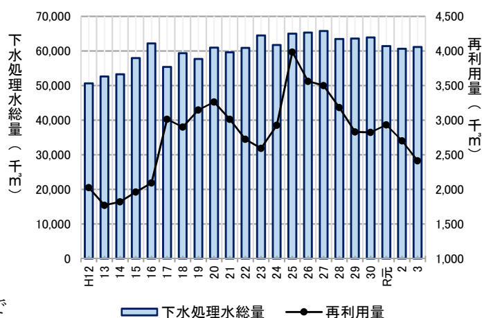
下水処理水再利用量の推移（場内および場外）
