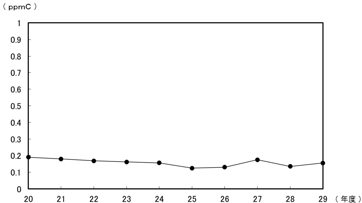
図 7 非メタン炭化水素濃度の推移 (測定局における 6~9 時年平均値の単純平均値の経年変化)
