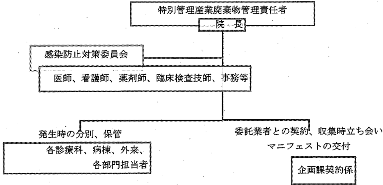
(管理体制図)
