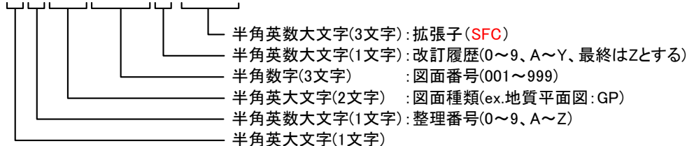
図 2-2 CAD データのファイル命名規則
