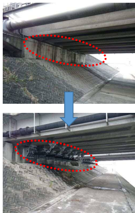
県道川津丸亀線(土器川大橋) 落橋防止装置による耐震化対策
