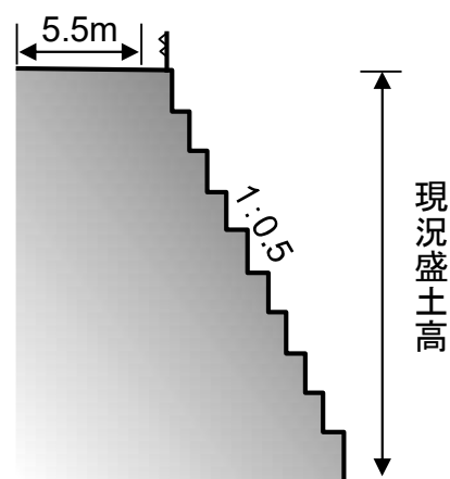
図 盛土法面の復旧イメージ
