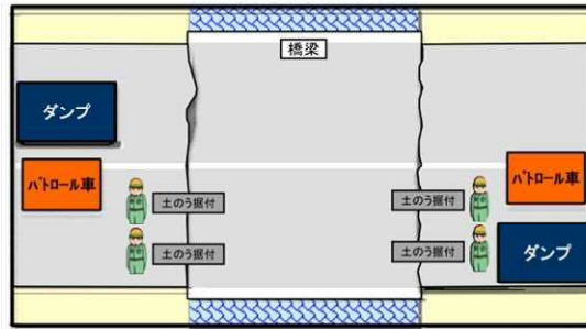
図 道路啓開の主な作業と必要資機材数（イメージ）
