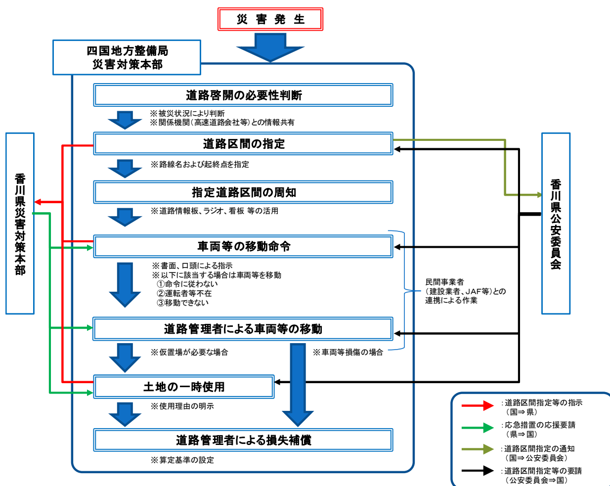
図 4-12 区間指定のフロー (国)
