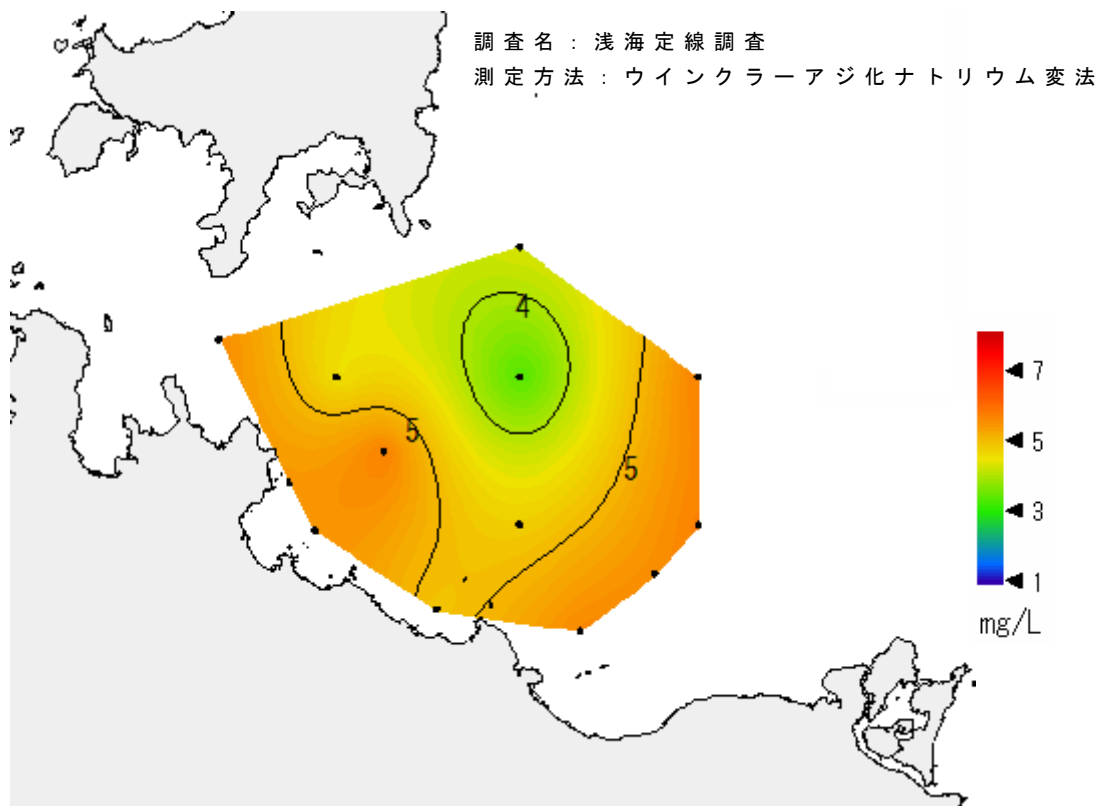
底層の溶存酸素濃度分布
