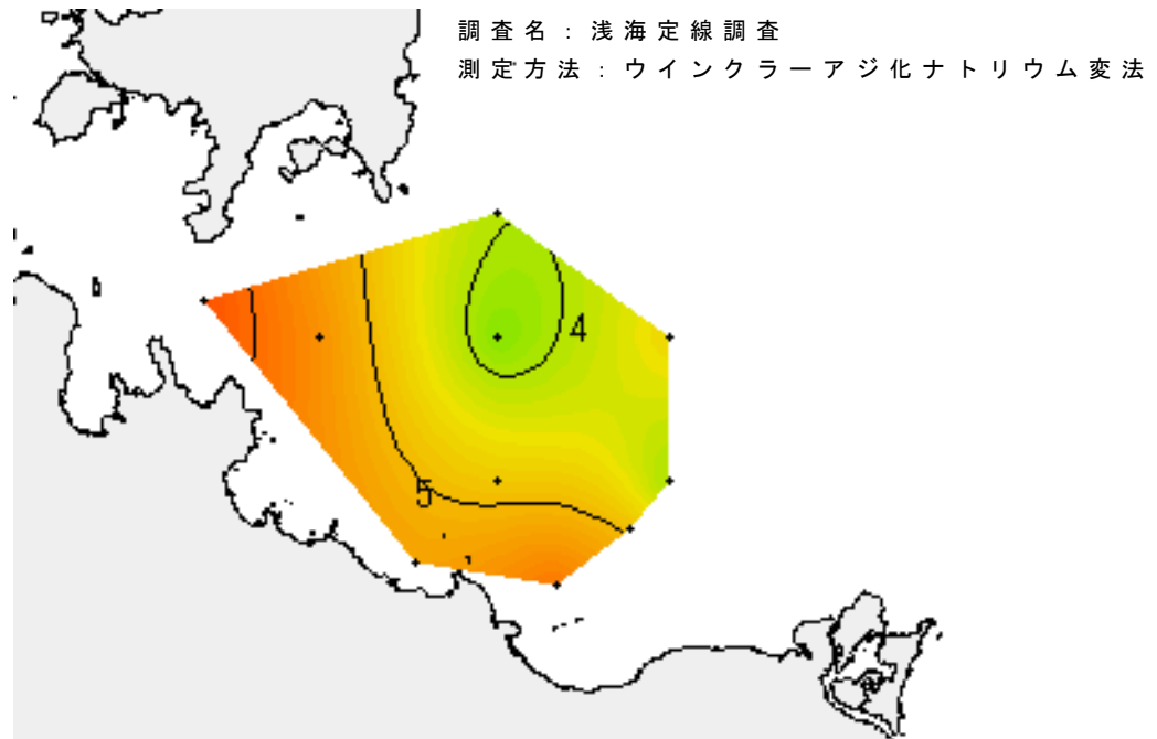
底層の溶存酸素濃度分布
