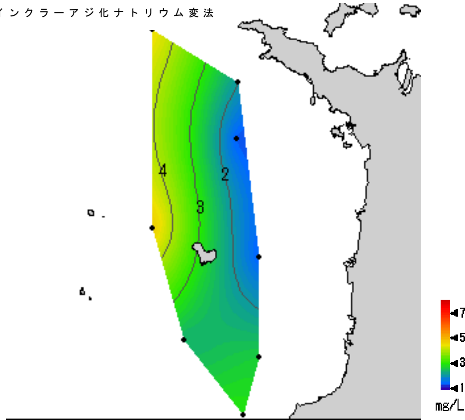
底層の溶存酸素濃度分布
