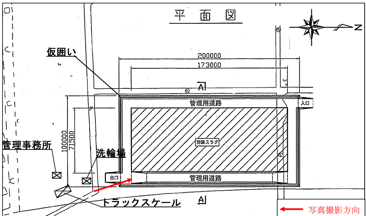
図1 平面図
