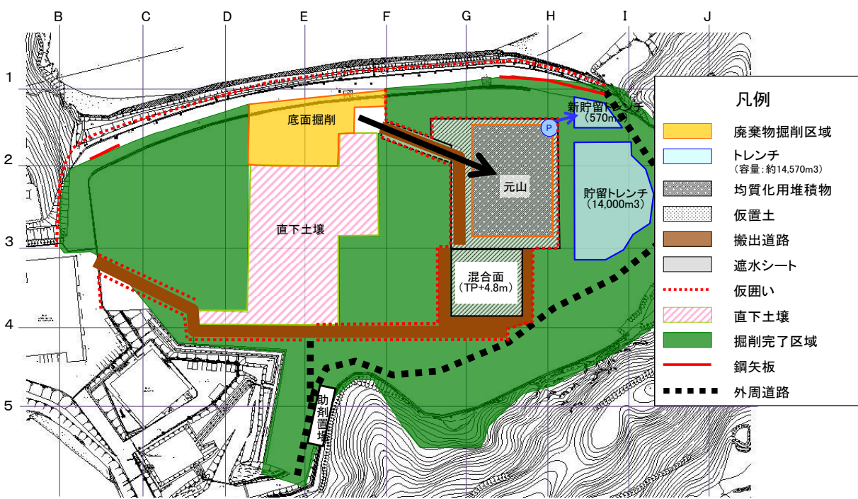
図2 平成28年12月掘削計画
