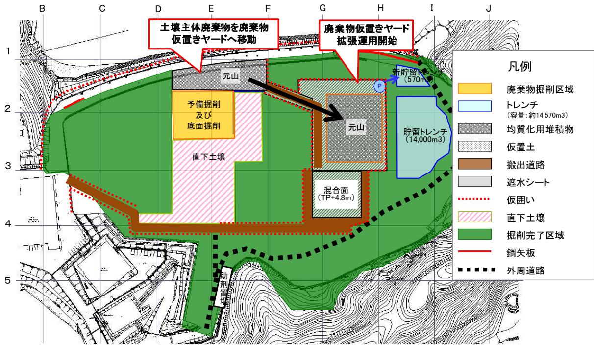
図1 平成28年11月掘削実績
