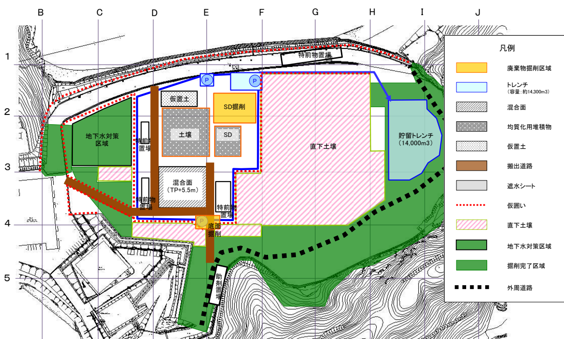
図2 平成27年11月掘削計画
