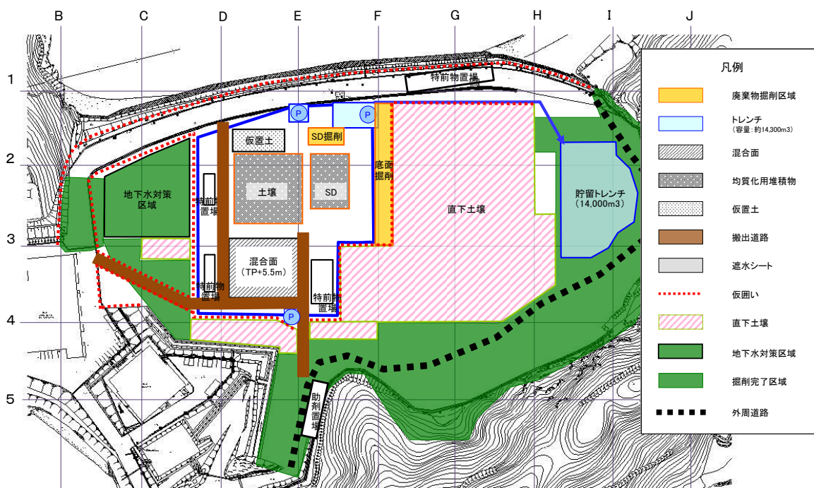
図1 平成27年10月掘削実績
