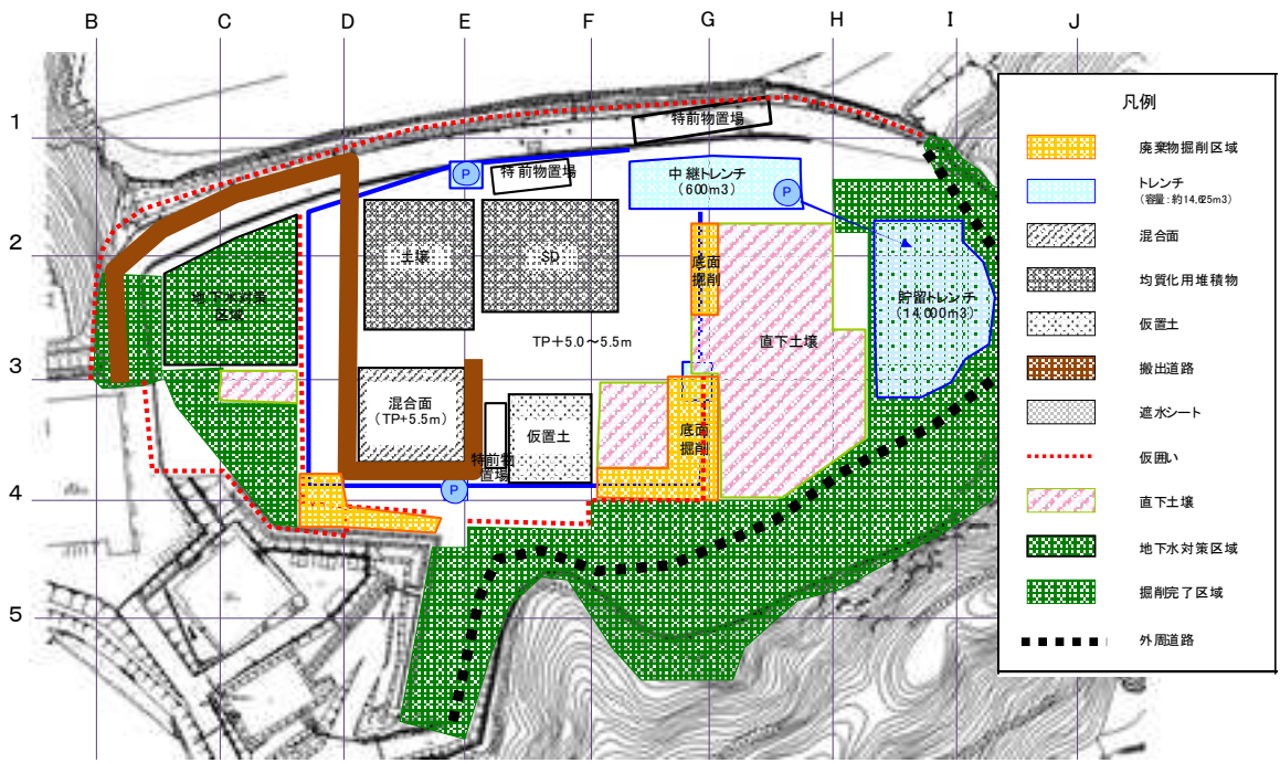
図2 平成27年2月掘削計画
