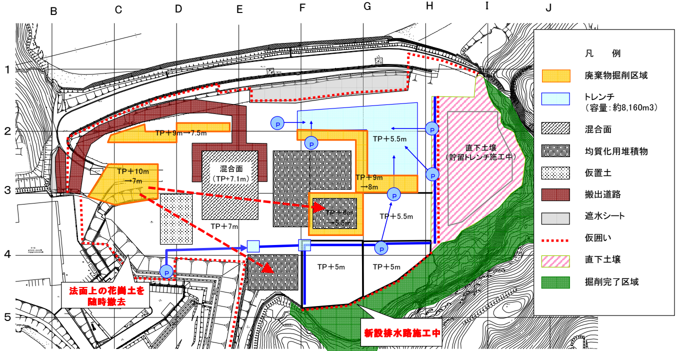
図1 平成25年1月掘削実績
