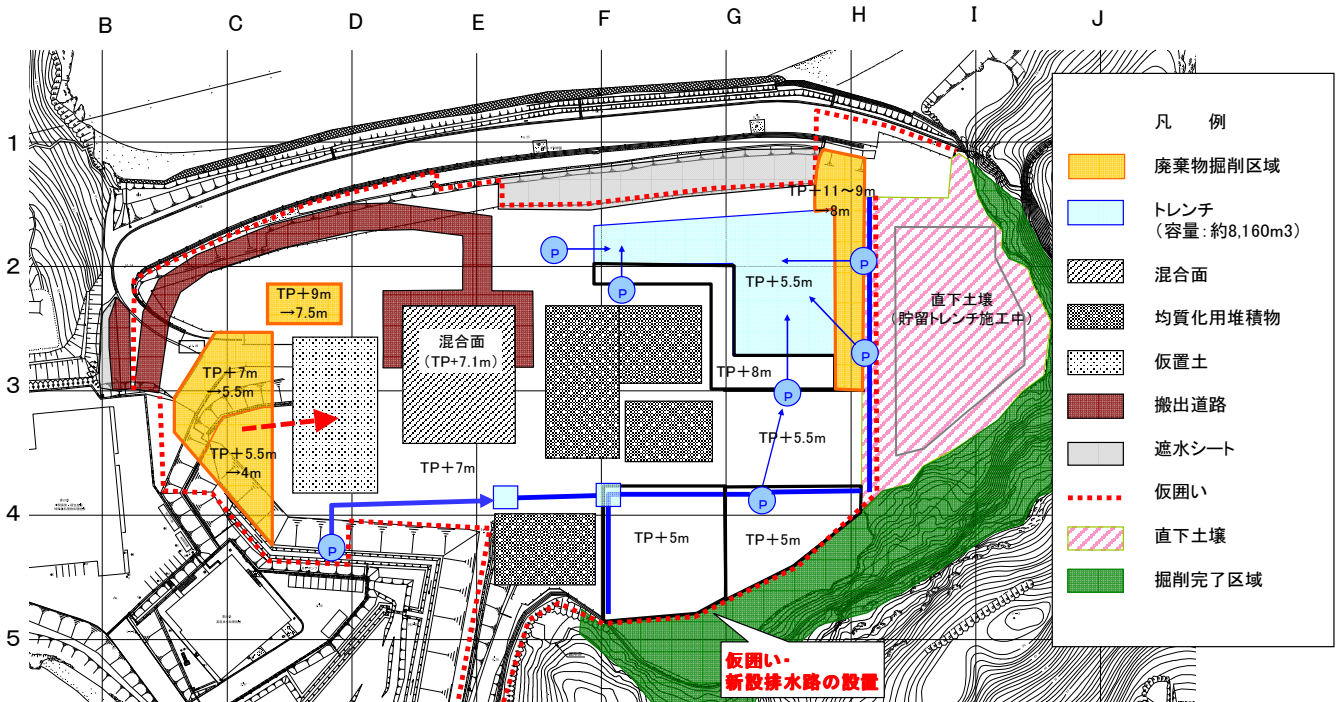
図2 平成25年2月掘削計画
