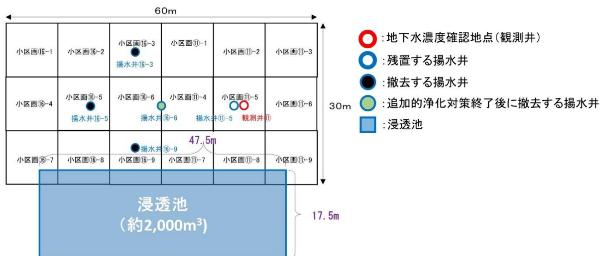
図5-2-3 HS-⑯における追加的浄化対策の状況 (R4.9.30 から追加的浄化対策を停止)
