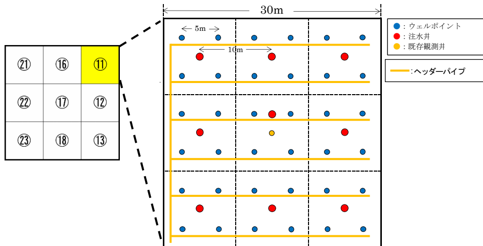
図3-3-2 各区画におけるウェルポイント等の平面配置
