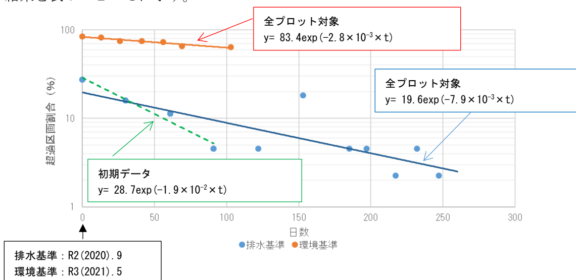
図7-2-2 始点からの排水基準及び環境基準の超過区画割合と各近似式
